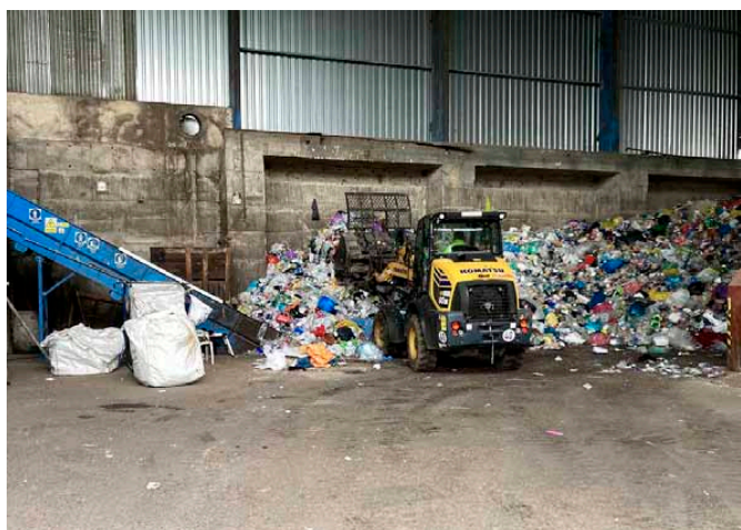
Návoz plastů do haly s dopravníkem
